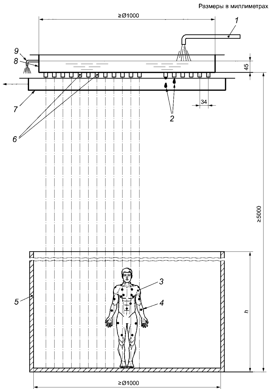
Рисунок 1 — Пример дождевой башни
